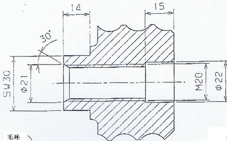
A-A 处剖面图
